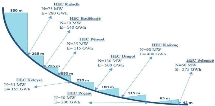
Skema e shfrytëzimit të Lumit Vjosa
