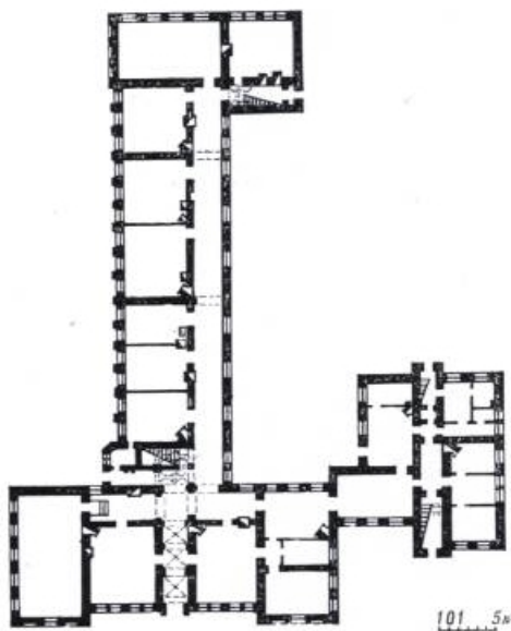
Мсціслаў. Будынак былой мужчынскай гімназіі. План першага паверха
