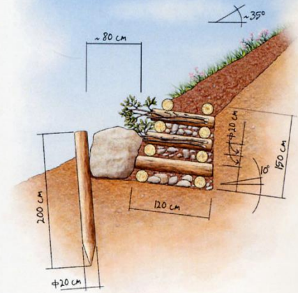
(b) Palo in legno
