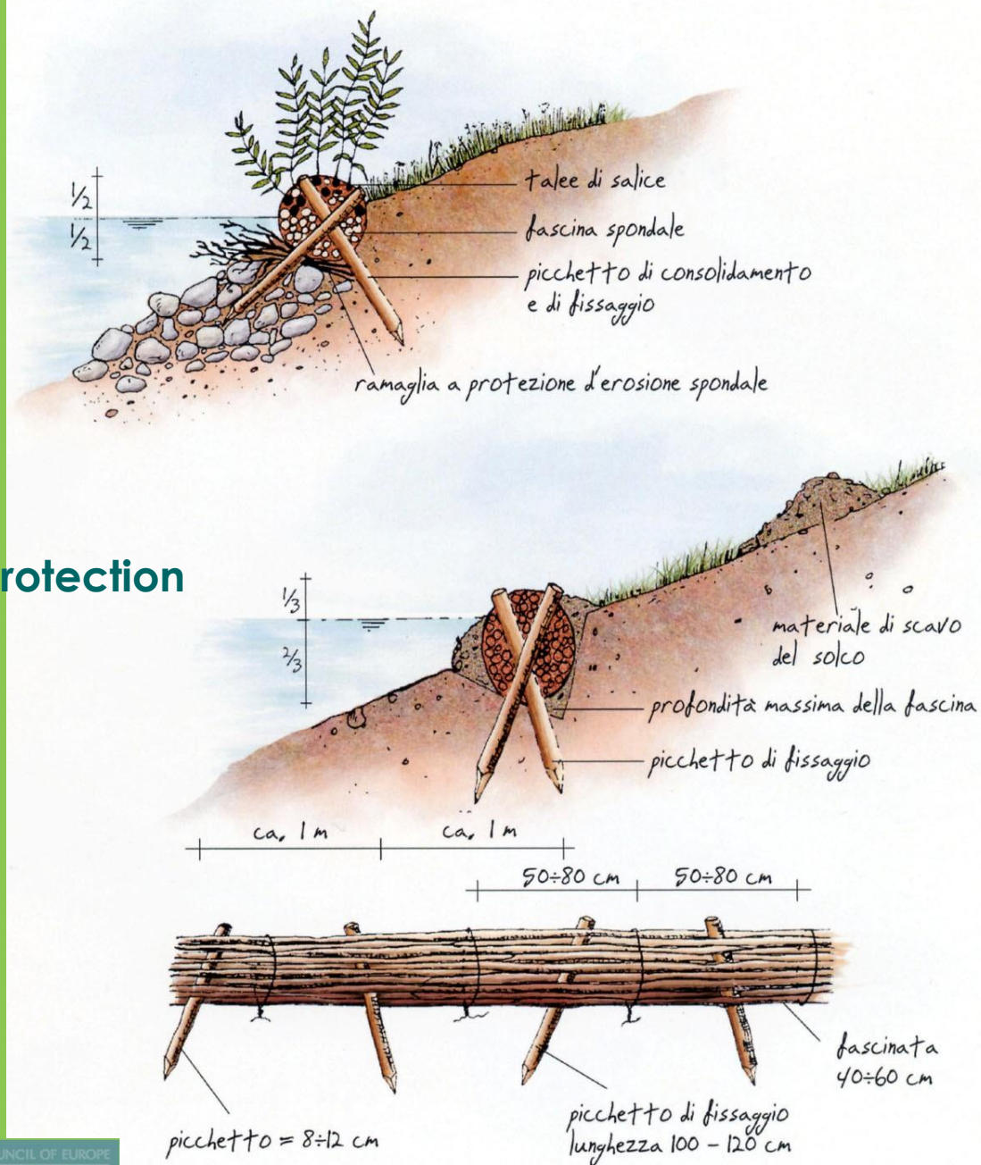
Figura 3.27: Fascinata viva spondale.
