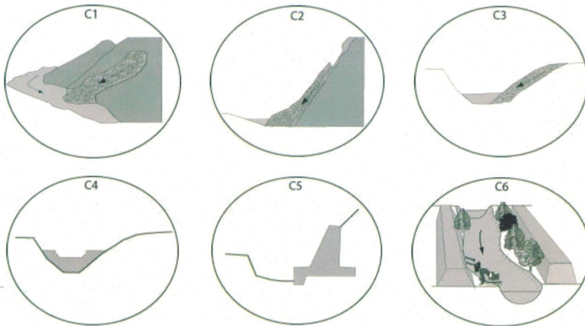
Figura 21 – Misure conservative. C1) non intervenire su frane; C2) non intervenire su versanti a diretto contatto con reticolo; C3) non intervenire su sponde in erosione; C4) non costruire nuove opere trasversali; C5) non costruire nuove opere longitudinali; C6) non fare manutenzione su opere esistenti.
