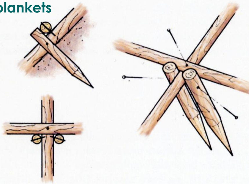
Figura 5.9: Predisposizione e fissaggio di una biorete.
