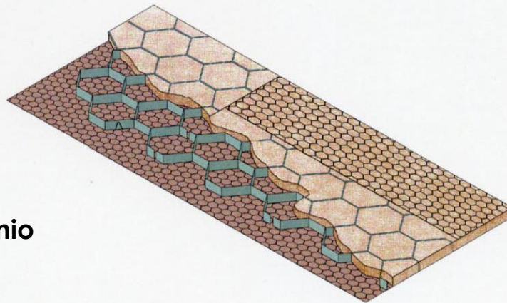
Figura 5.12: Geocelle costituite di strisce di geotessile apribili a fisarmonica.
