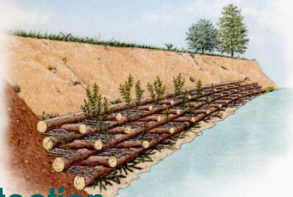
(a) Palificata viva spondale ad una parete
