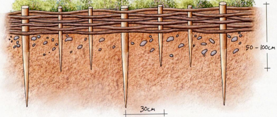
Figura 3.23: Intreccio alternato di materiale vegetale vivo.
