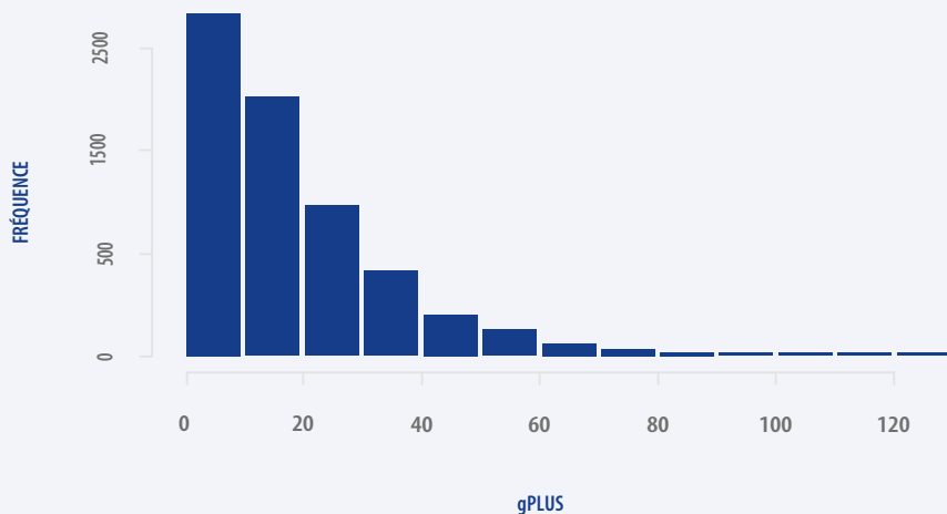
Figure 2.16 – Distribution des erreurs de Guttman – Bloc 4.1
