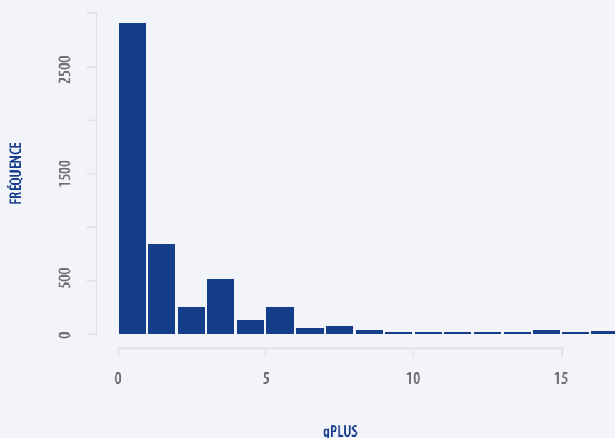
Figure 2.4 – Distribution des erreurs de Guttman – Bloc 2
