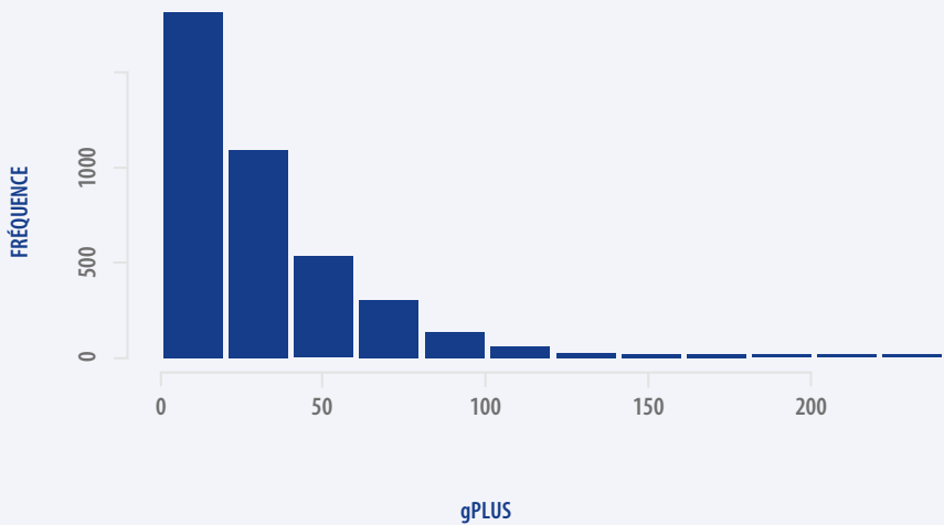
Figure 2.36 – Distribution des erreurs de Guttman – Bloc 5.2
