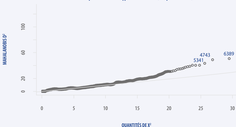
Figure 2.19 – Diagramme quantile-quantile de Mahalanobis D^2 en fonction des quantiles du \chi^2 – Bloc 4.2 (importance)
