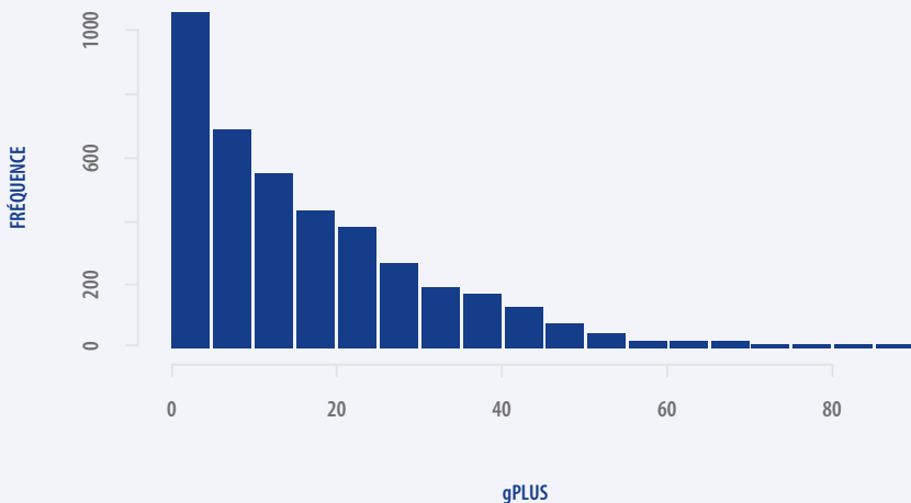
Figure 2.28 – Distribution des erreurs de Guttman – Bloc 4.3
