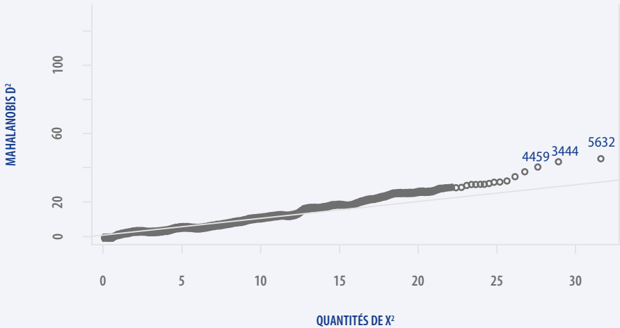
Figure 2.15 – Diagramme quantile-quantile de Mahalanobis D 2 en fonction des quantiles du χ 2 – Bloc 4.1
