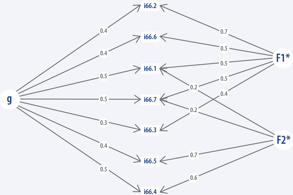
Figure 2.25 – Modèle de mesure – Bloc 4.2 (fréquence)
