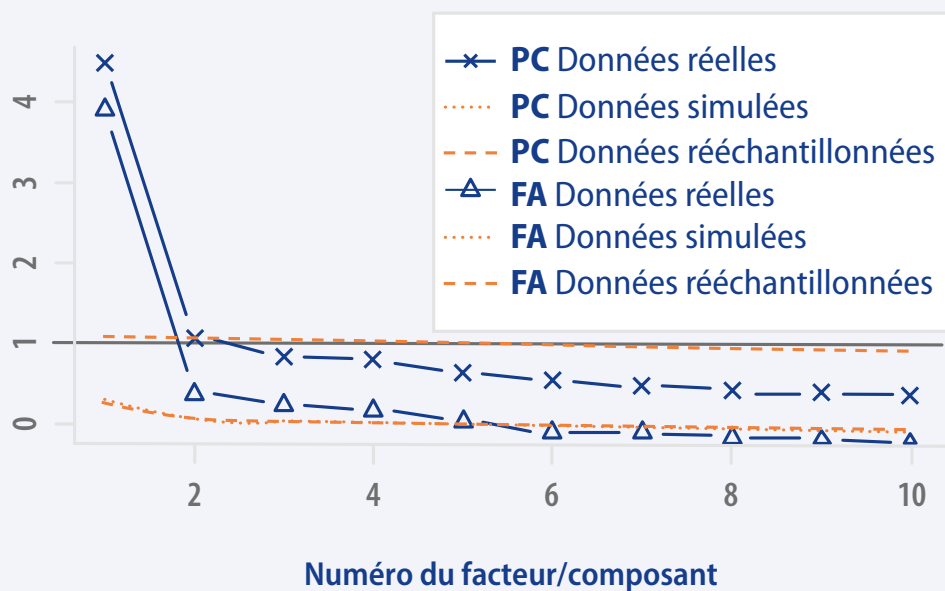
Figure 2.38 – Graphique de sédimentation – Bloc 5.2
