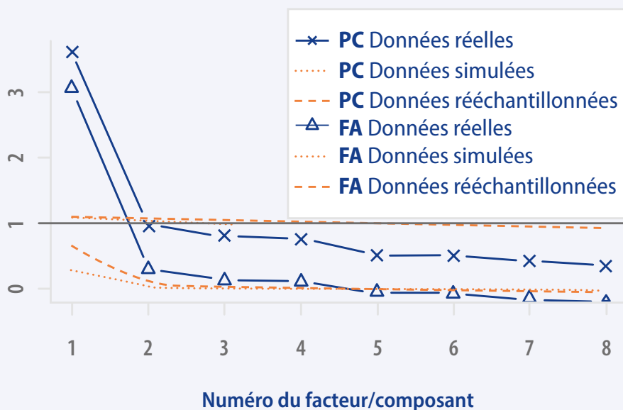
Figure 2.22 – Graphique de sédimentation – Bloc 4.2 (importance)
