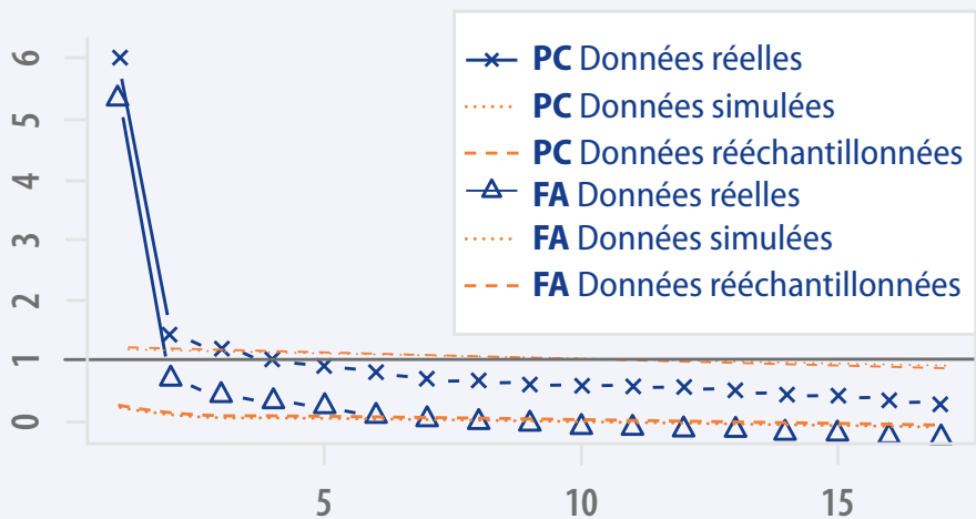
Figure 2.10 – Graphique de sédimentation – Bloc 3.1
