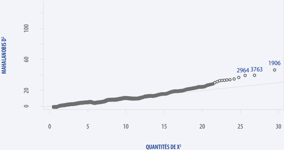
Figure 2.23 – Diagramme quantile-quantile de Mahalanobis D^2 en fonction des quantiles du \chi^2 – Bloc 4.2 (fréquence)
