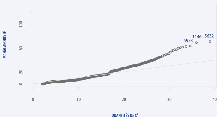
Figure 2.11 – Diagramme quantile-quantile de Mahalanobis D 2 en fonction des quantiles du \chi^2 – Bloc 3.2
