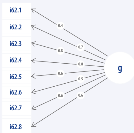
Figure 2.17 – Modèle de mesure – Bloc 4.1
