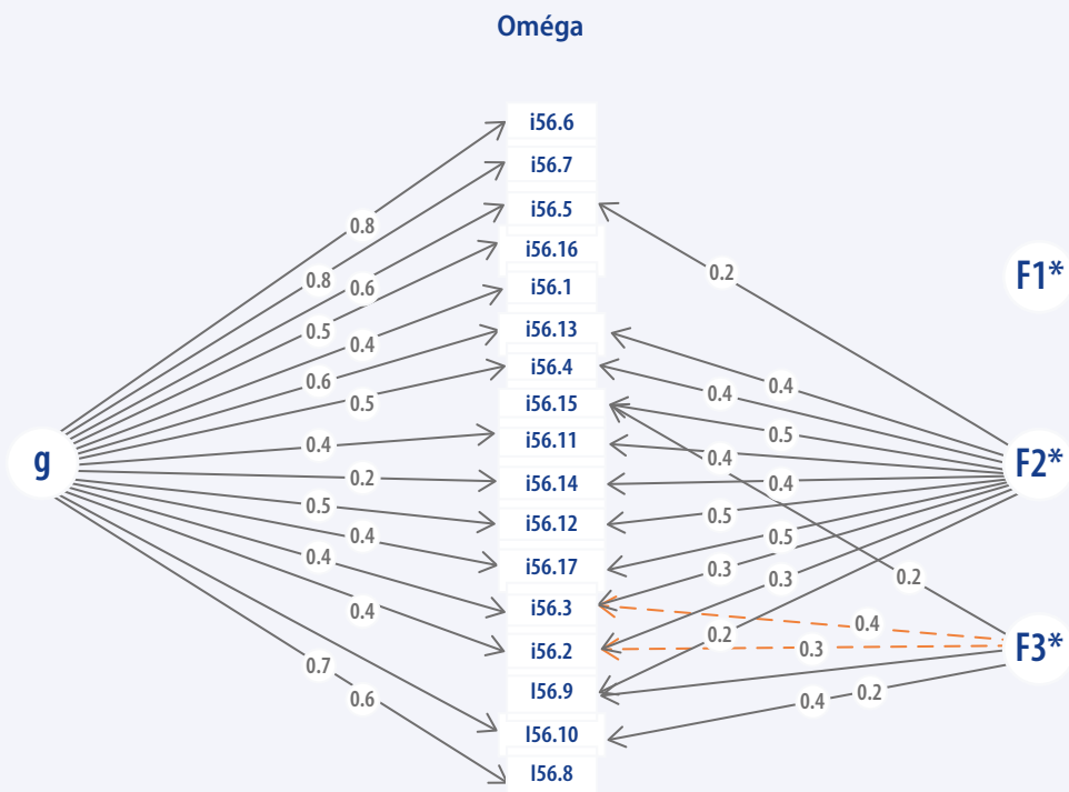
Figure 2.9 – Modèle de mesure – Bloc 3.1
