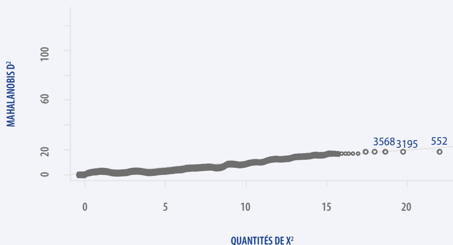
Figure 2.3 – Diagramme quantile-quantile de Mahalanobis D^2 en fonction des quantiles du \chi^2 – Bloc 2
