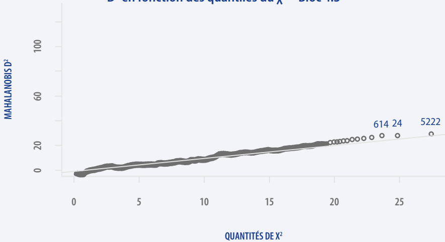
Figure 2.27 – Diagramme quantile-quantile de Mahalanobis D^2 en fonction des quantiles du \chi^2 – Bloc 4.3
