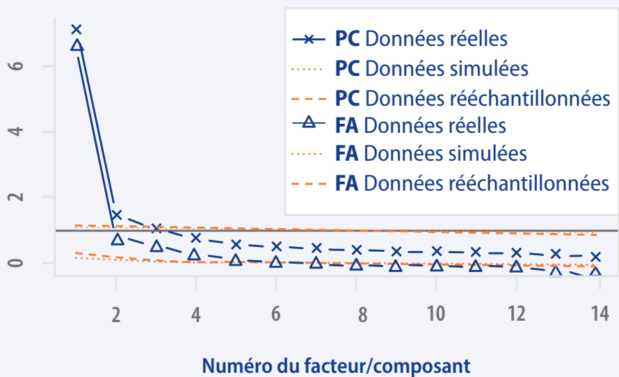
Figure 2.34 – Graphique de sédimentation – Bloc 5.1
