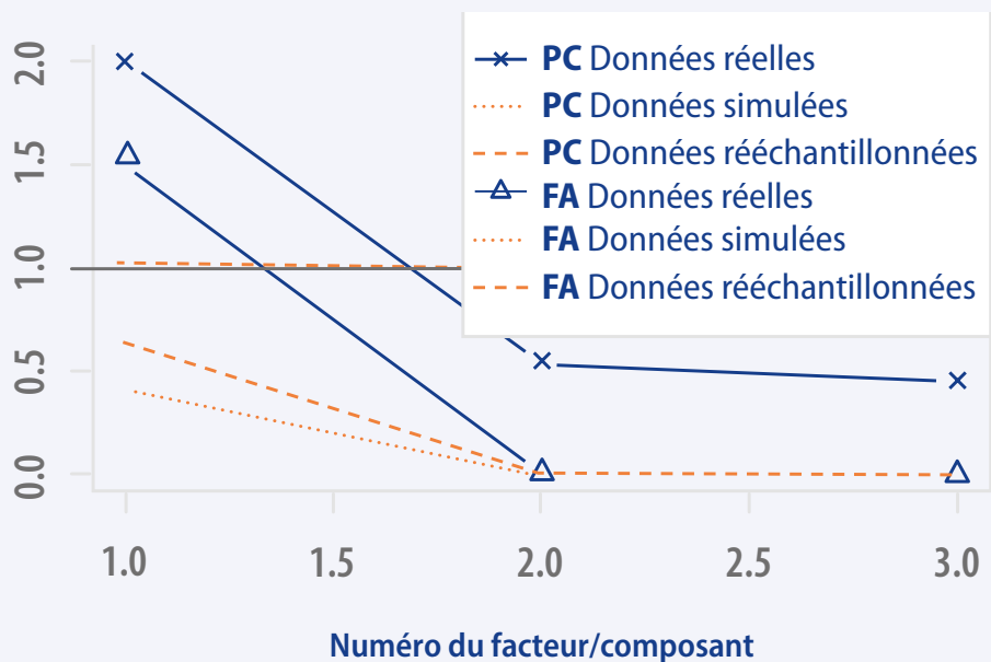
Figure 2.6 – Graphique de sédimentation – Bloc 2
