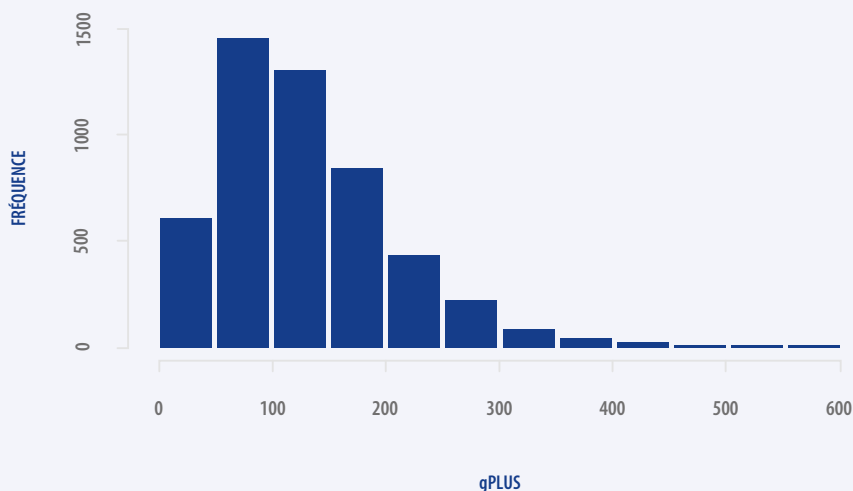
Figure 2.8 – Distribution des erreurs de Guttman – Bloc 3.1
