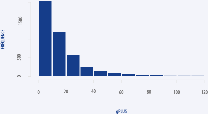
Figure 2.24 – Distribution des erreurs de Guttman – Bloc 4.2 (fréquence)
