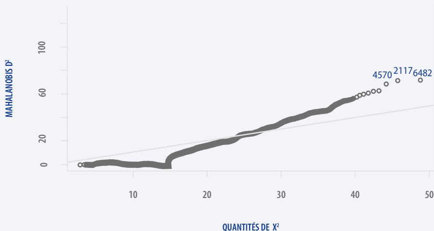
Figure 2.7 – Diagramme quantile-quantile de Mahalanobis D^2 en fonction des quantiles du \chi^2 – Bloc 3.1
