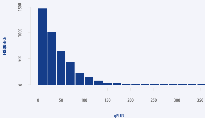
Figure 2.32 – Distribution des erreurs de Guttman – Bloc 5.1
