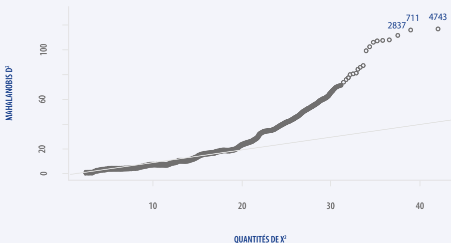
Figure 2.31 – Diagramme quantile-quantile de Mahalanobis D 2 en fonction des quantiles du \chi^2 – Bloc 5.1
