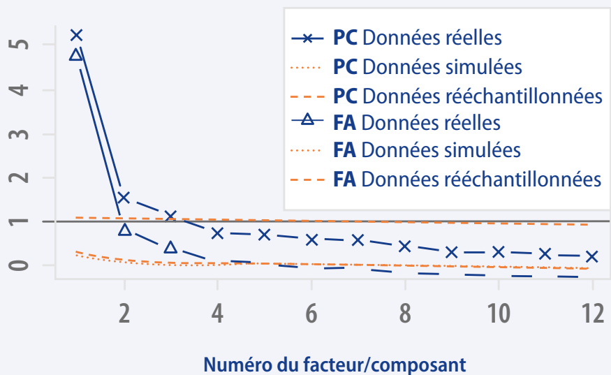
Figure 2.14 – Graphique de sédimentation – Bloc 3
