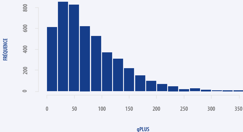
Figure 2.12 – Distribution des erreurs de Guttman – Bloc 3.2
