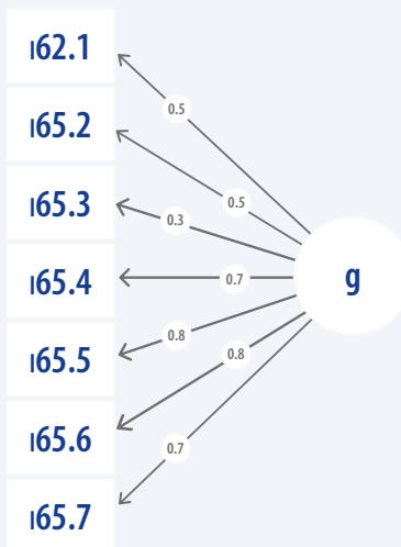
Figure 2.21 – Modèle de mesure – Bloc 4.2 (importance)
