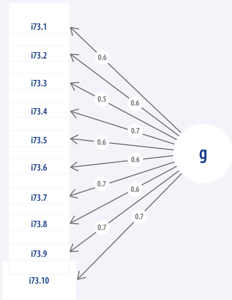
Figure 2.37 – Modèle de mesure – Bloc 5.2
