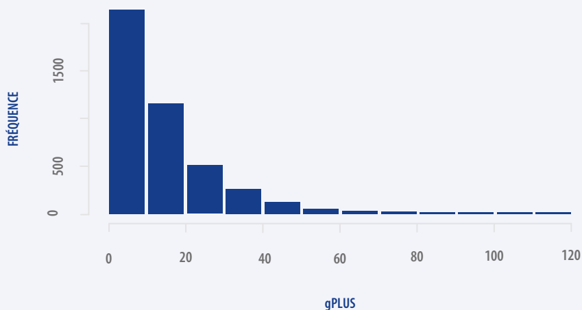
Figure 2.20 – Distribution des erreurs de Guttman – Bloc 4.2 (importance)
