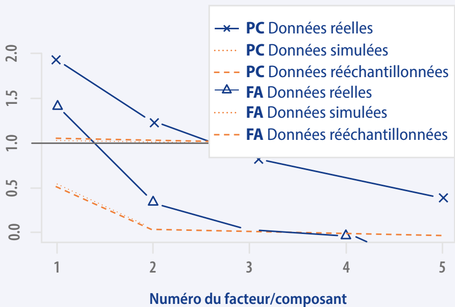
Figure 2.30 – Graphique de sédimentation – Bloc 4.3
