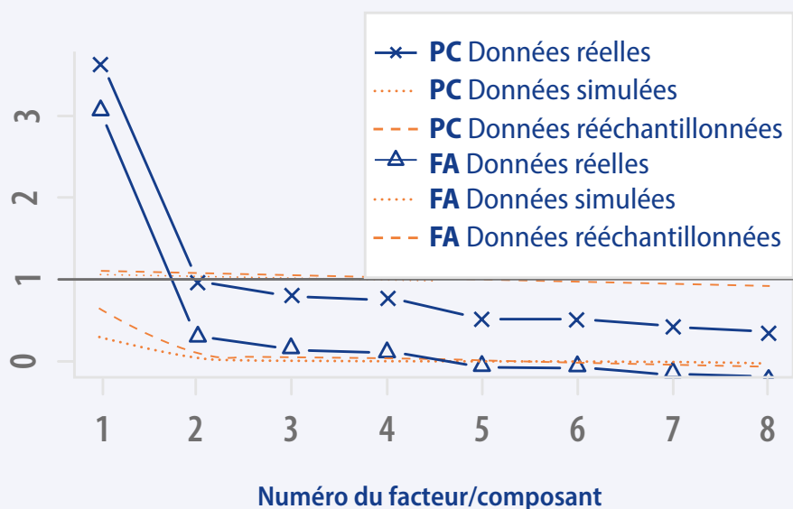
Figure 2.18 – Graphique de sédimentation – Bloc 4.1
