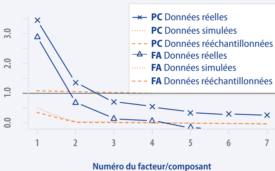
Figure 2.26 – Graphique de sédimentation – Bloc 4.2 (fréquence)
