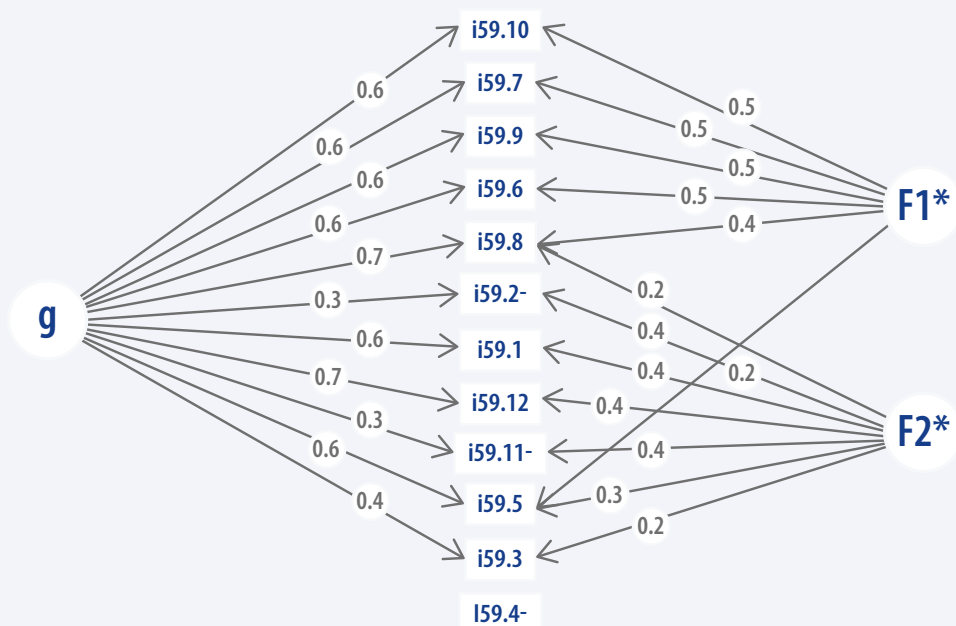
Figure 2.13 – Modèle de mesure – Bloc 3.2
